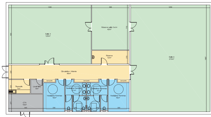
Plan provisoire en phase d'avant-projet sommaire.
