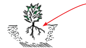
JEUNES SUJETS : 50-60cm de diamètre et de profondeur GROS SUJETS : 1m de diamètre et 0.80m de profondeur
