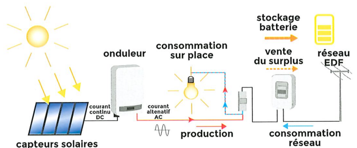
Installation photovoltaïque alliant consommation sur place et revente du surplus
