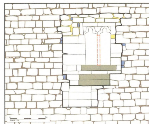
Etat II Etat III Blocs de remplis ? Restitution du meneau Blocs de calage (insertion ?)
