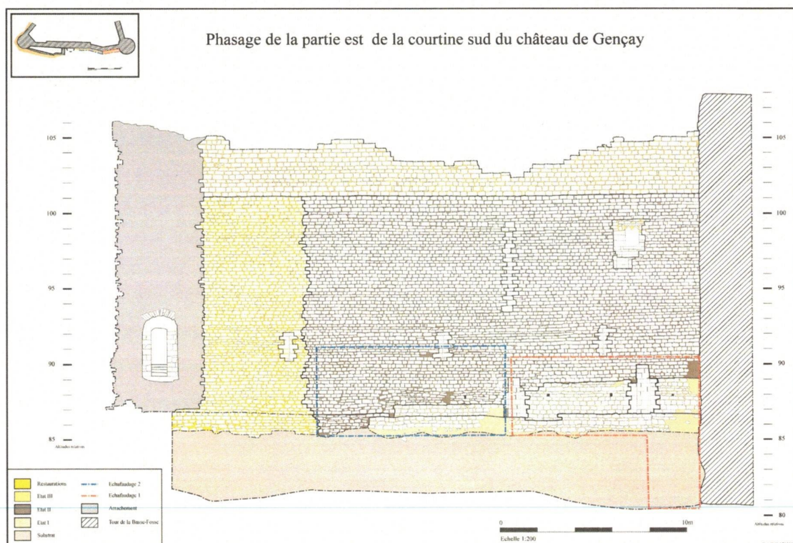
Fig. 2 : Dessin Assisté par Ordinateur (D.A.O) des différentes phases de construction de la courtine (D.A.O. C. ARMAND©)
