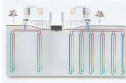
Système de PAC sur Géothermie verticale
