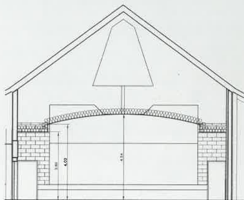
COUPE GRANDE SALLE
