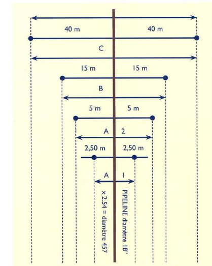
ZONE DE RISQUES (pipeline diamètre 457)
