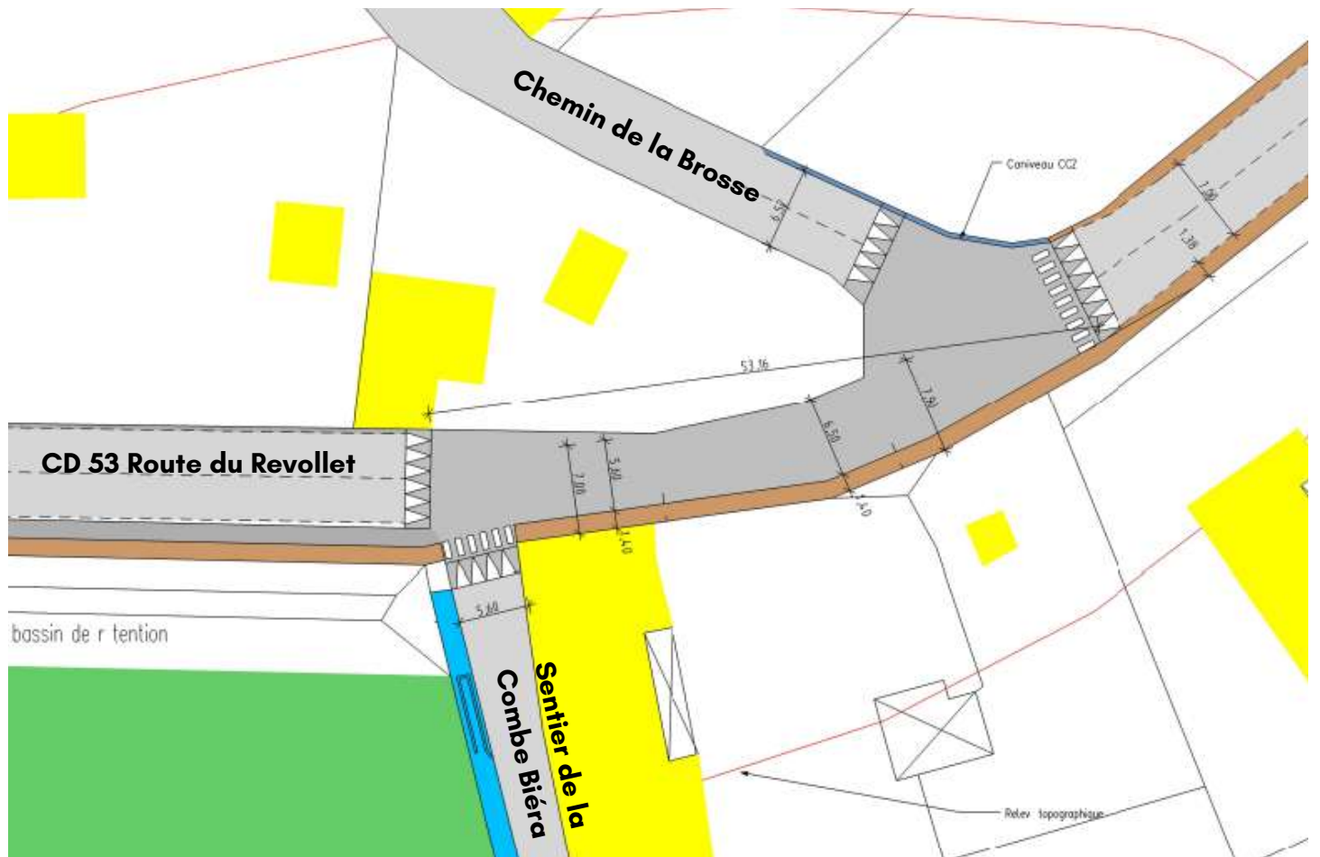
Plateau ralentisseur au carrefour chemin de la Brosse
