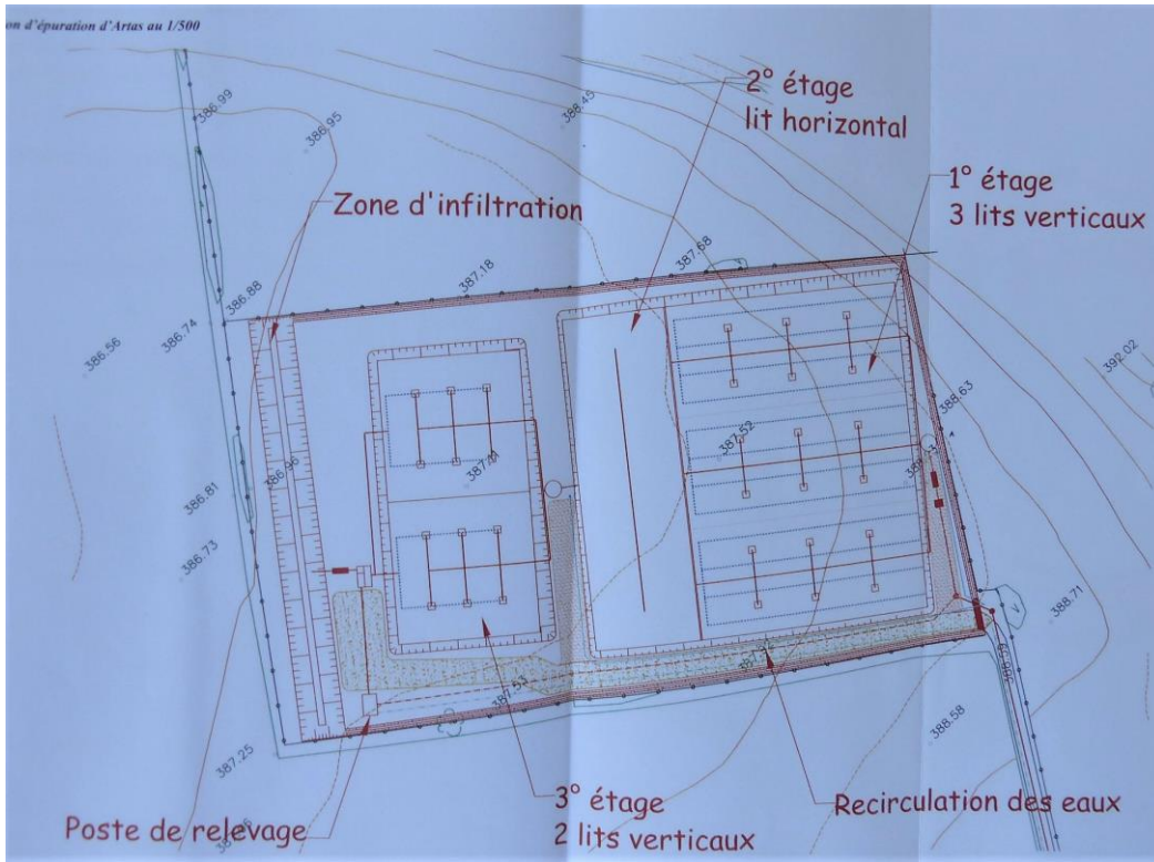
Schéma de fonctionnement de la station d'épuration
