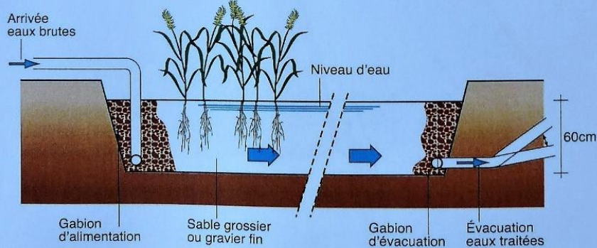
FILTRE HORIZONTAL : ALIMENTATION CONTINUE
