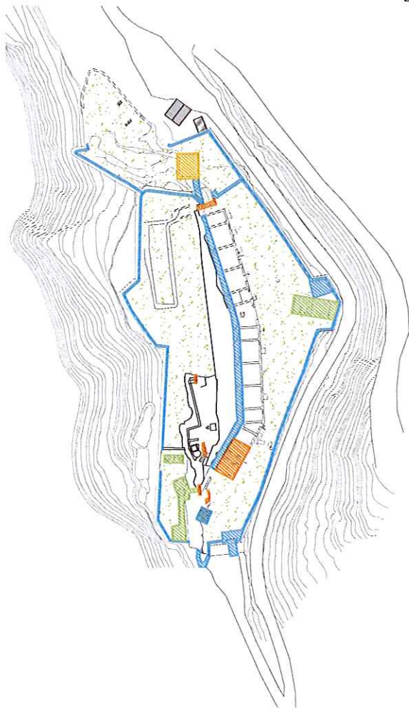
PLAN DU R+1 DE LA REDOUTE RUINÉE
