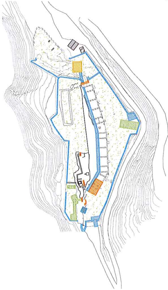
PLAN DU R+1 DE LA REDOUTE RUINÉE 0 2 4 20m
