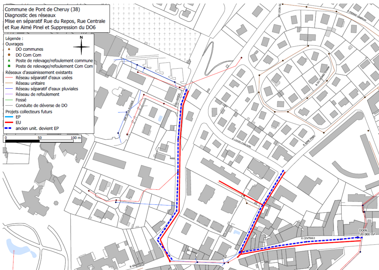
Figure 20 : Mise en séparatif en amont du DO6
