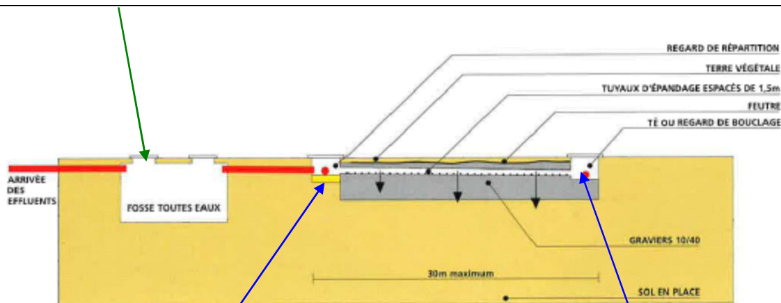
Coupe longitudinale : schéma de principe
