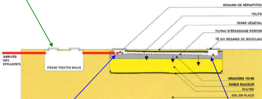
Coupe longitudinale : schéma de principe
