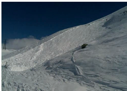
Avalanche au col de la Traversette en mars 2011
