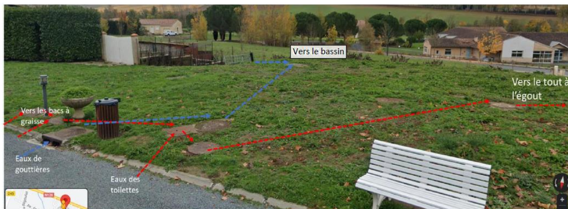
Schéma des réseaux de collecte
