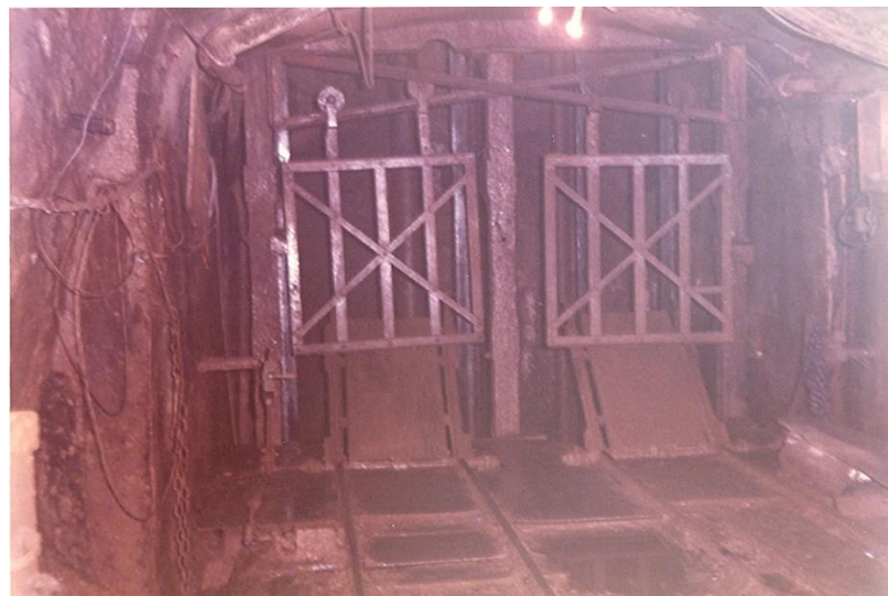
Figure 26 : Les berlines transportant le minerai et les cages du puits reliant le sous-sol à la surface
