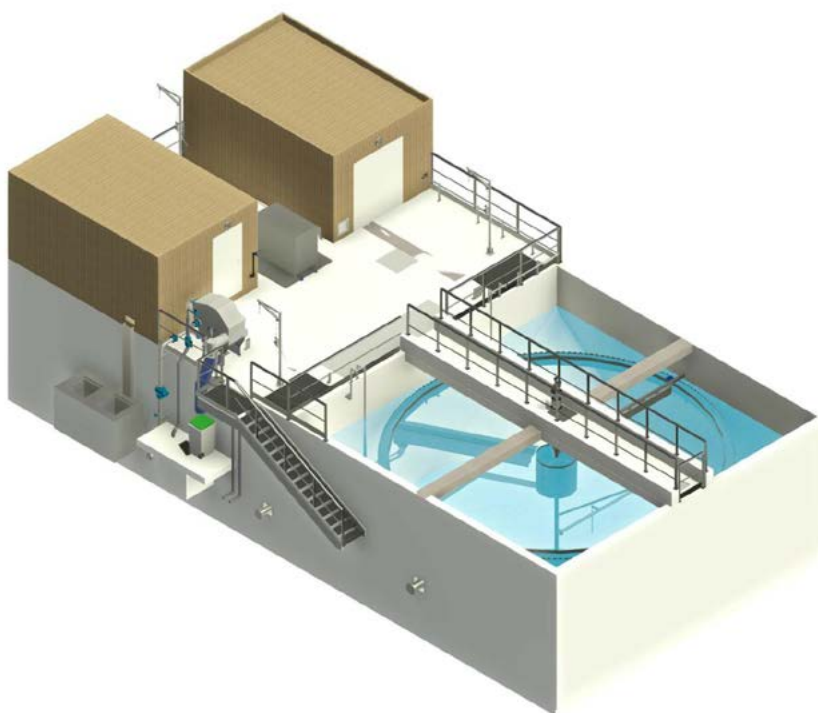
Bassin d'aération.
