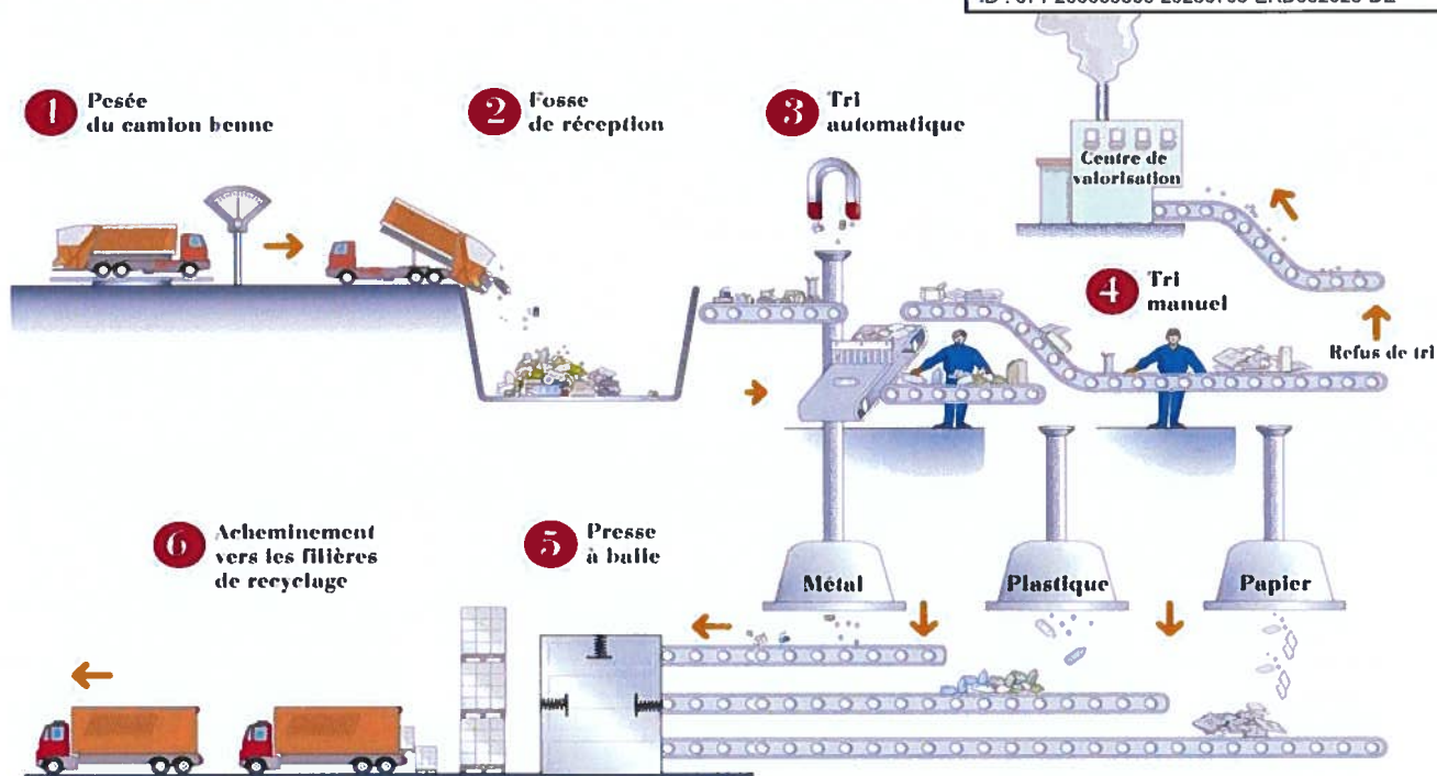
Figure 8 : Schéma de fonctionnement d'un centre de tri
