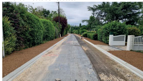
Travaux route de Beausseuil
