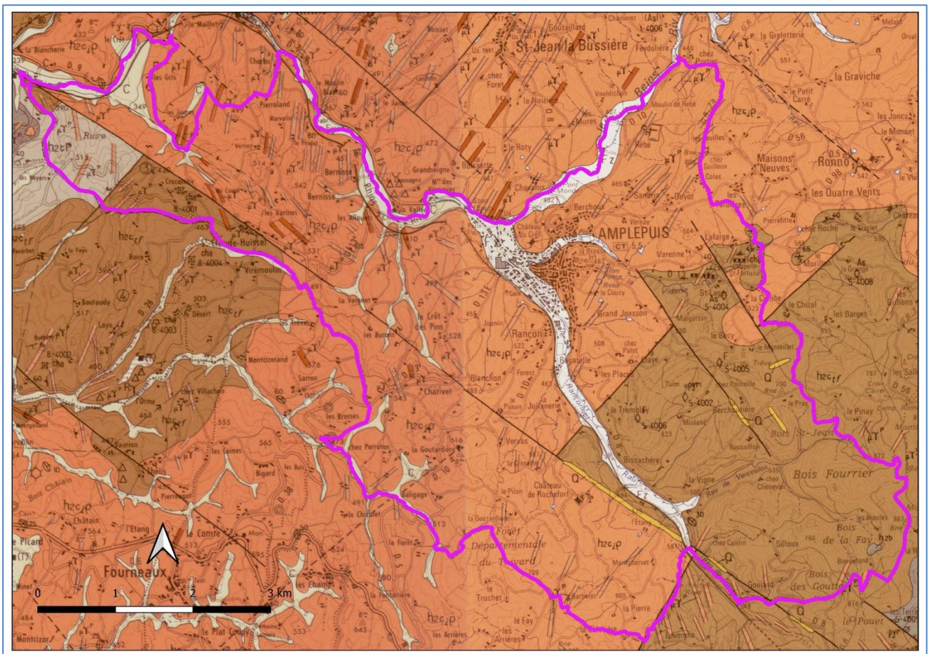
Figure 2 : carte géologique de la commune d'AMPLEPUIS (1/50000)
