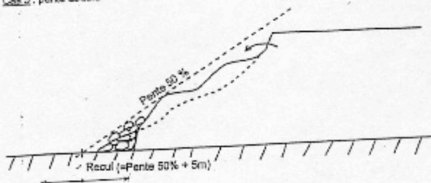
Cas 5 : pente double
