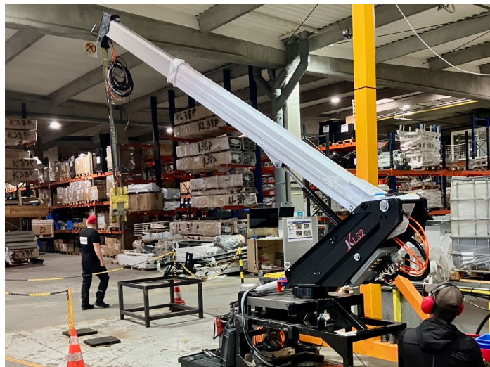
Test d'un bras articulé avant son montage sur véhicule dans l'atelier de Ferrières-en-Brie
