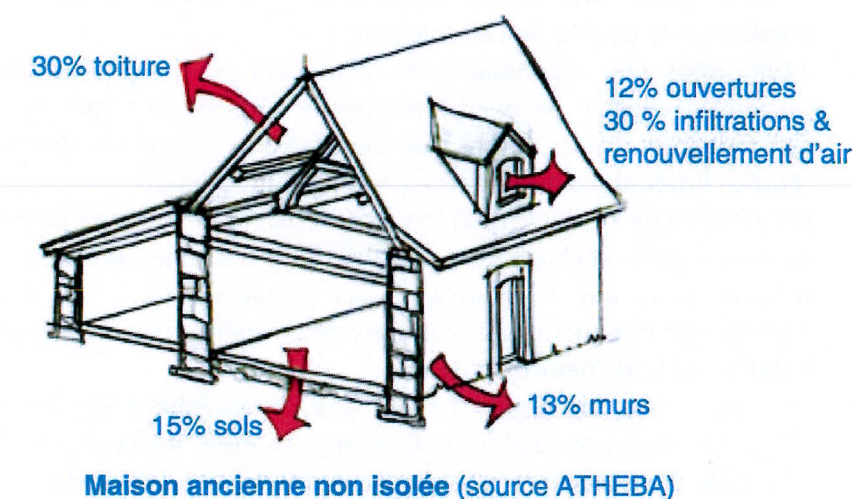
Proportions moyennes des déperditions d'un bâtiment non isolé [Source : ATHEBA]
