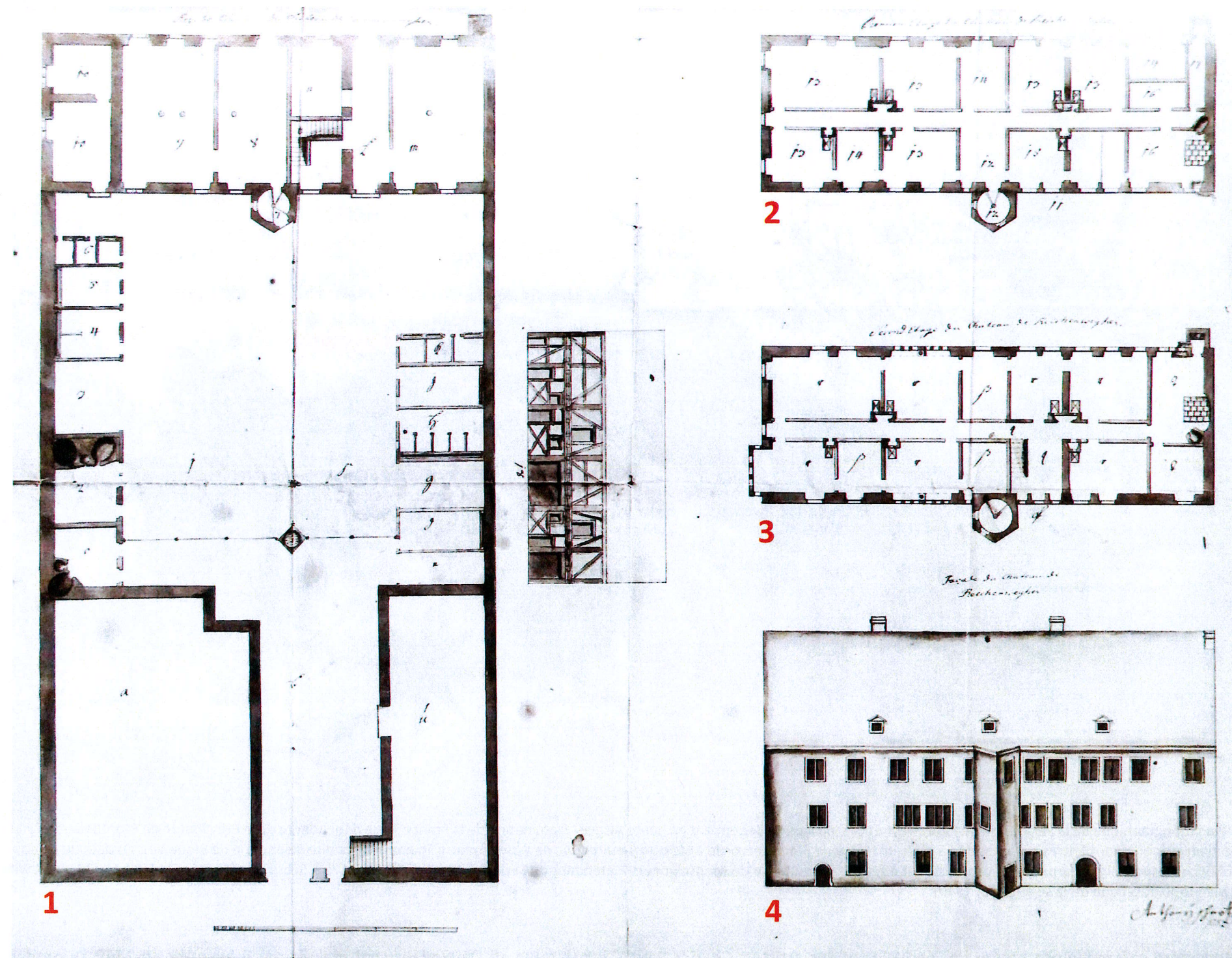
1 : « Rez-de-chaussée du château de Reichenweyer » ; 2 : « Premier étage du château de Reichenweyer » ; 3 : « Second étage du château de Reichenweyer » ; 4 : « Façade du château de Reinchenweyer », signé Anthony Schrotz, 1752 [Source: AAC, 1 Fi 389, Riquewihr : plan du château , 1752]
