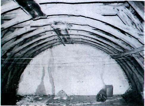
Détails de la charpente en berceau et de l'assemblage des arbalétriers et des aisseliers, 1344 [Source : MPP, E/81/68/31_11, ancienne chapelle de l'hôpital St-Erard, ph : J-P. Beck, 1983]
