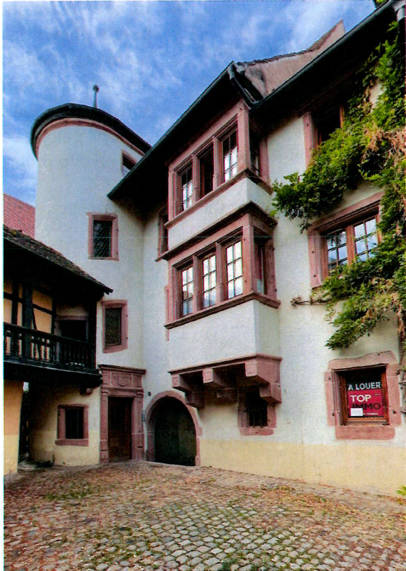
Oriel à deux niveaux, cour de Strasbourg [Source : AFK, 2024]
