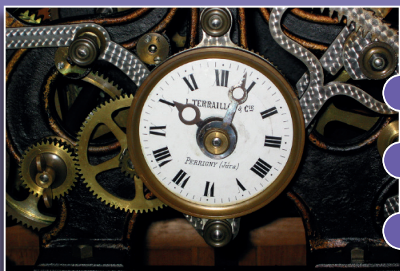
Ancien mécanisme de l'horloge de la mairie
