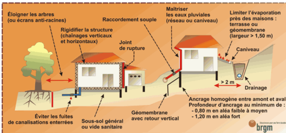
Schéma de synthèse des dispositions préventives
