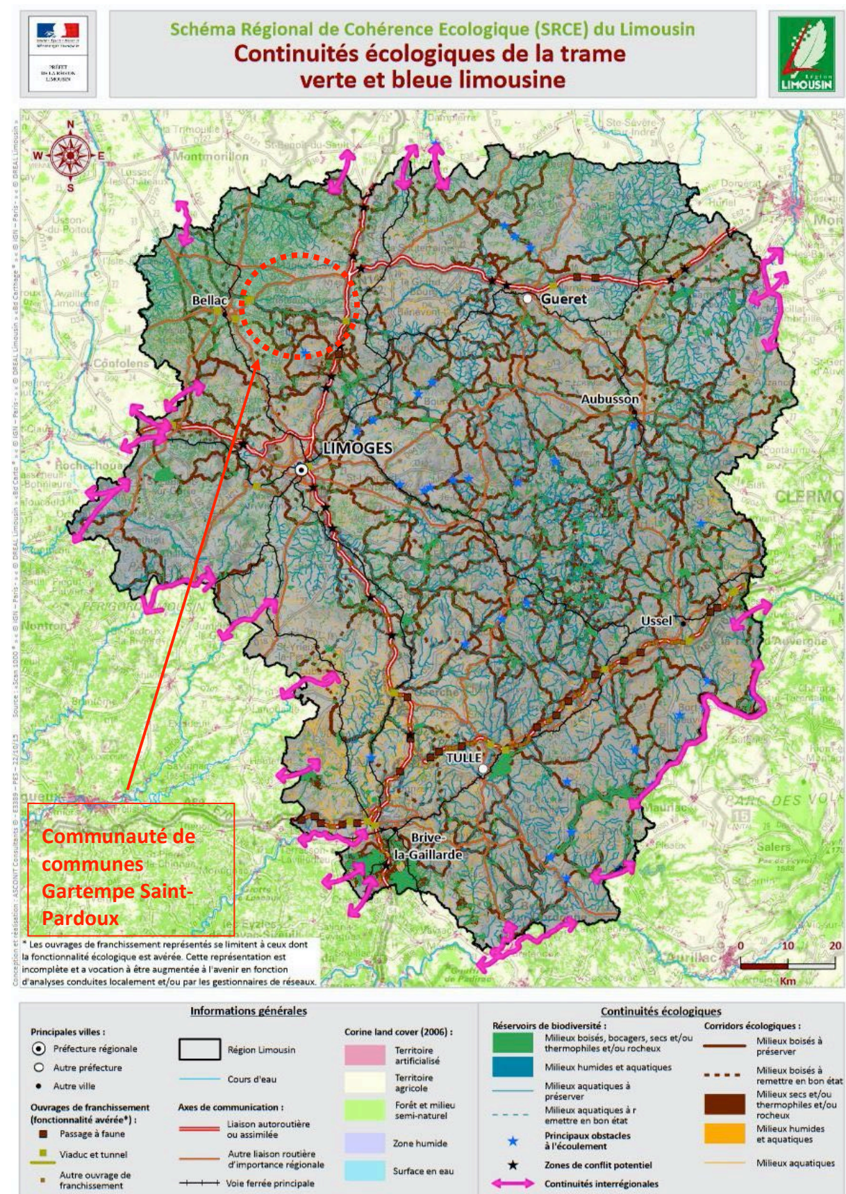
Figure 28 : Schéma Régional de Cohérence Ecologique du Limousin : Continuité écologique de la trame verte et bleue limousine Source : SRCE Limousin, Région Limousin, ASCONIT Consultant
