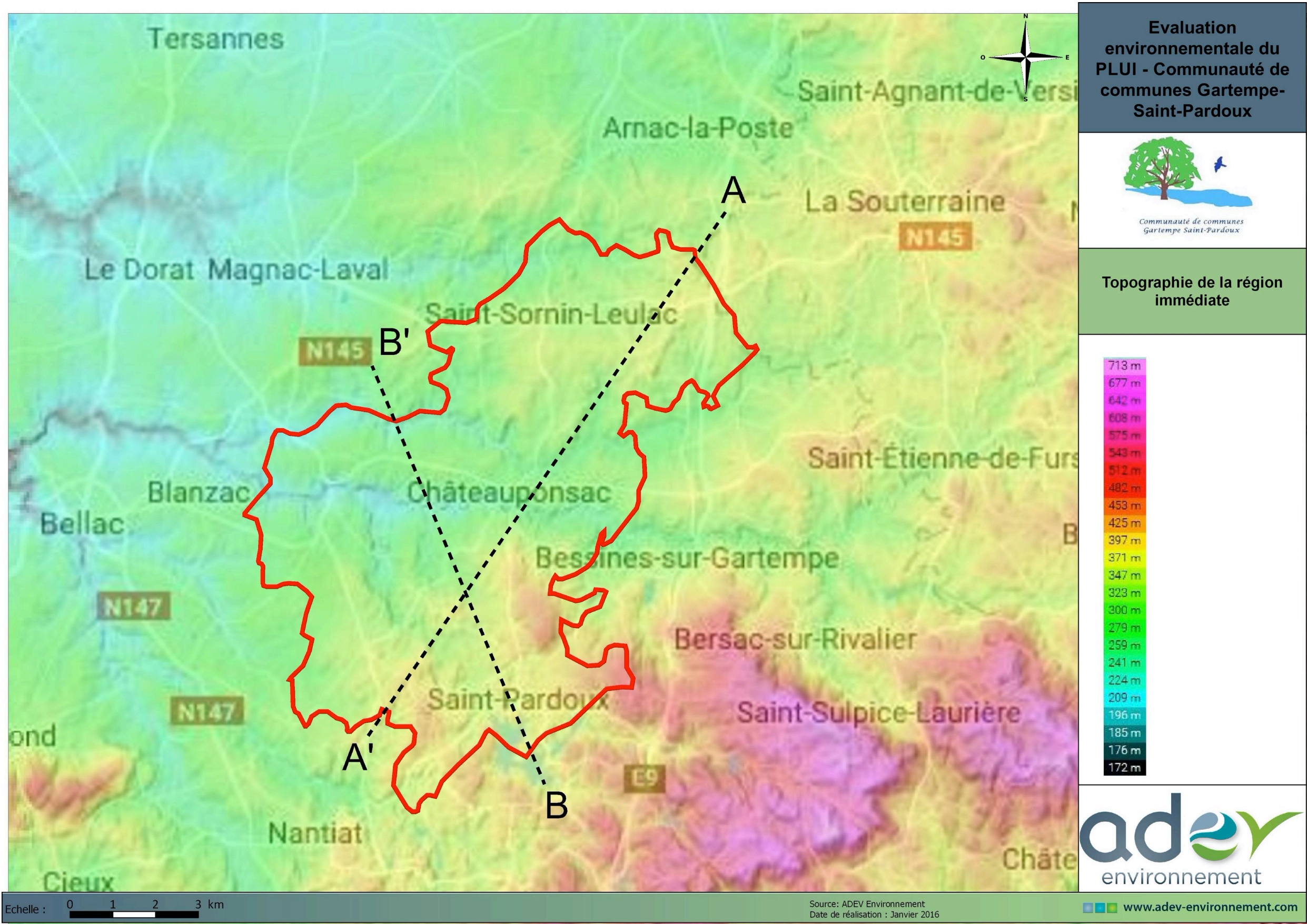
Figure 3 : Topographie de la région immédiate de la Communauté de communes Gartempe Saint-Pardoux (Source : Topographic-map)
