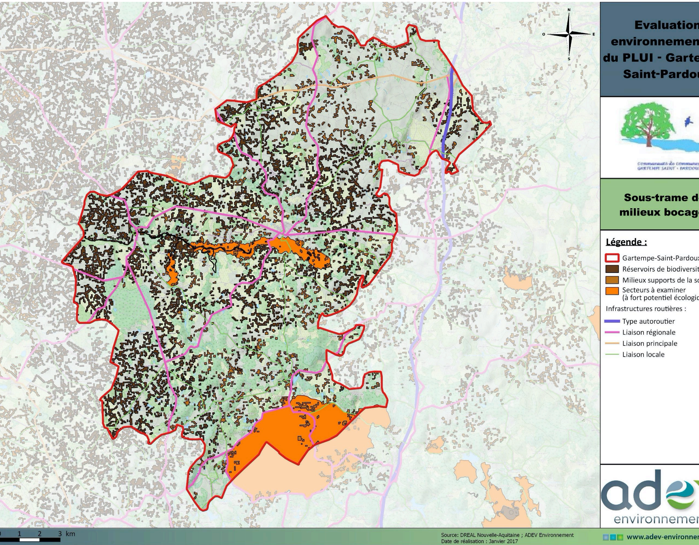
Figure 29 : SRCE Limousin : Sous-trame des milieux bocagers (Source : SRCE Limousin)
