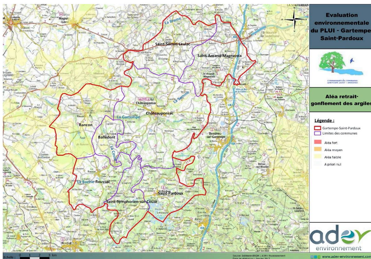
Figure 93 : Le retrait-gonflement des argiles
