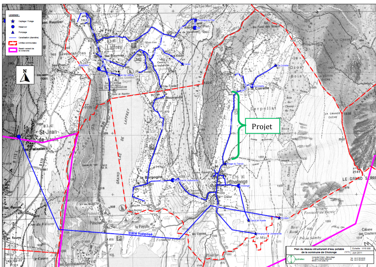
Réseaux AEP source : Schéma directeur des eaux potables, HYDRATEC, 2011
