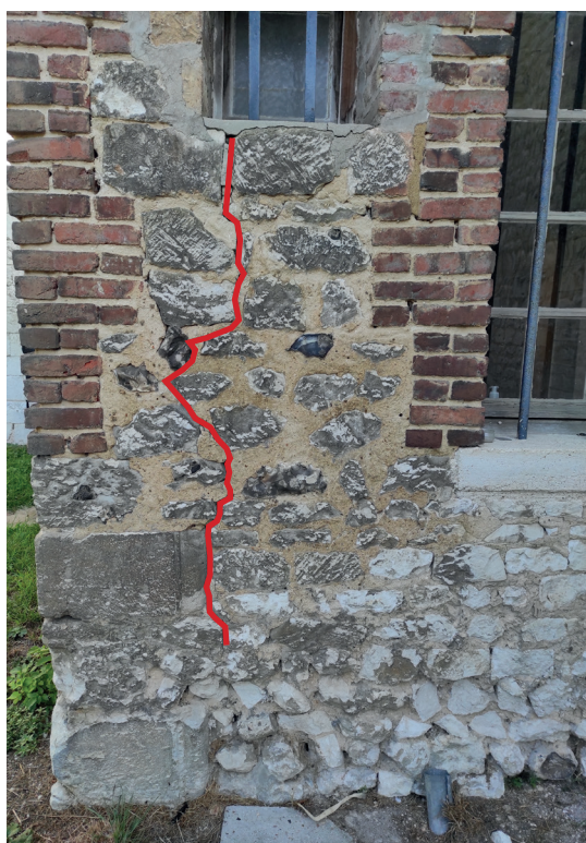
9. Sacristie, fissure désolidarisant l'angle.
