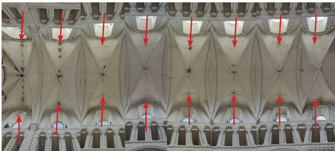
12. Voûtes du vaisseau principal de la nef, fissures dites de Sabouret traduisant un déliaisonnement continu avec les gouttereaux, réseau de micro-fissures.
