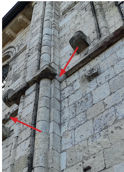
4. Bandeau présentant des pierres cassées voire manquantes. Érosion refuge sous la corniche, présence accrue de nids et traces d'anciens aujourd'hui enlevées.
