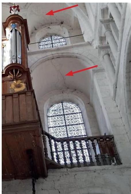
20. Prolongement des fissurations en appui de la tribune d'orgue dans les parties hautes.
