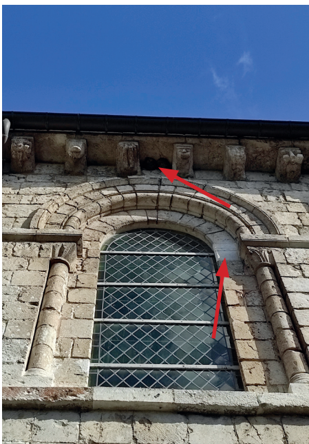
4. Nidification entre les modillons, pierres de remplacement très marquées.
