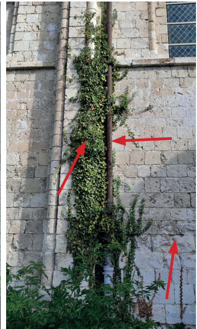
3. Contrefort largement envahi sous des plantes grimpantes, descente de gouttière fortement envahie. Érosion des pierres.
