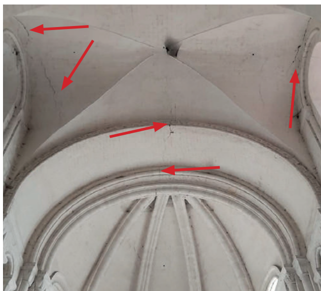
17. Fissuration longitudinale de l'arc doubleau se prolongeant jusque dans l'abside et fissure dite de Sabouret au droit des voûtes.
