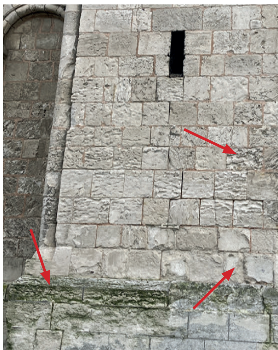
12. Développements importants de micro-végétaux sur les reliefs, desquamation et érosion de la pierre.
