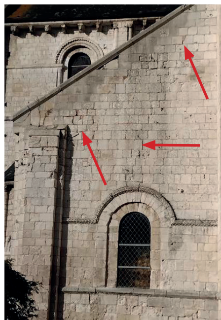
16. Fissurations verticales: ouvertures des joints en escalier.
