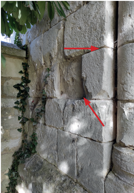
1. Développement de plantes grimpantes, perte importante de matière et déjointoiement des pierres.
