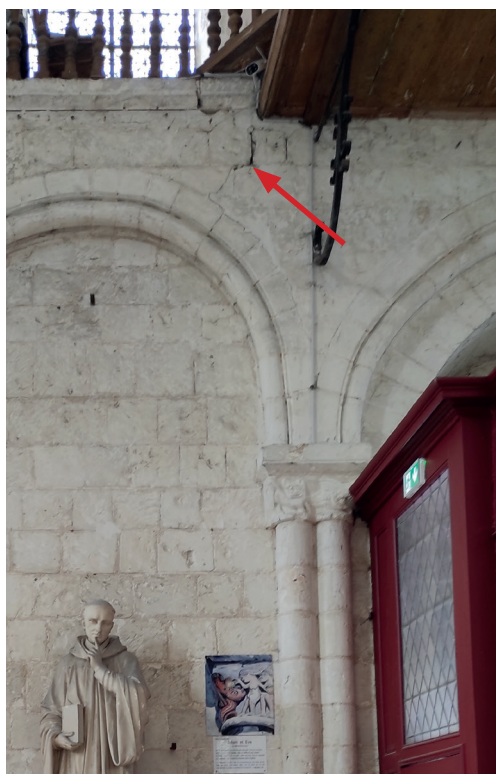
18. Fissures au droit de l'appui de la tribune d'orgue.
