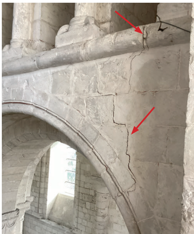
15. Fissuration verticale du tas de charge et fissuration des claveaux de l'arc.
