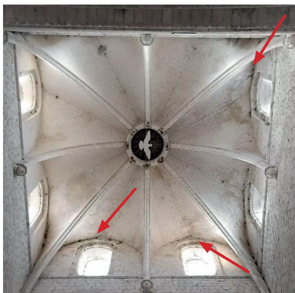
16. Fissures dites de Sabouret: anciennes ?.
