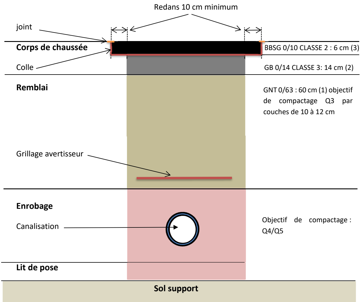
Schéma type
