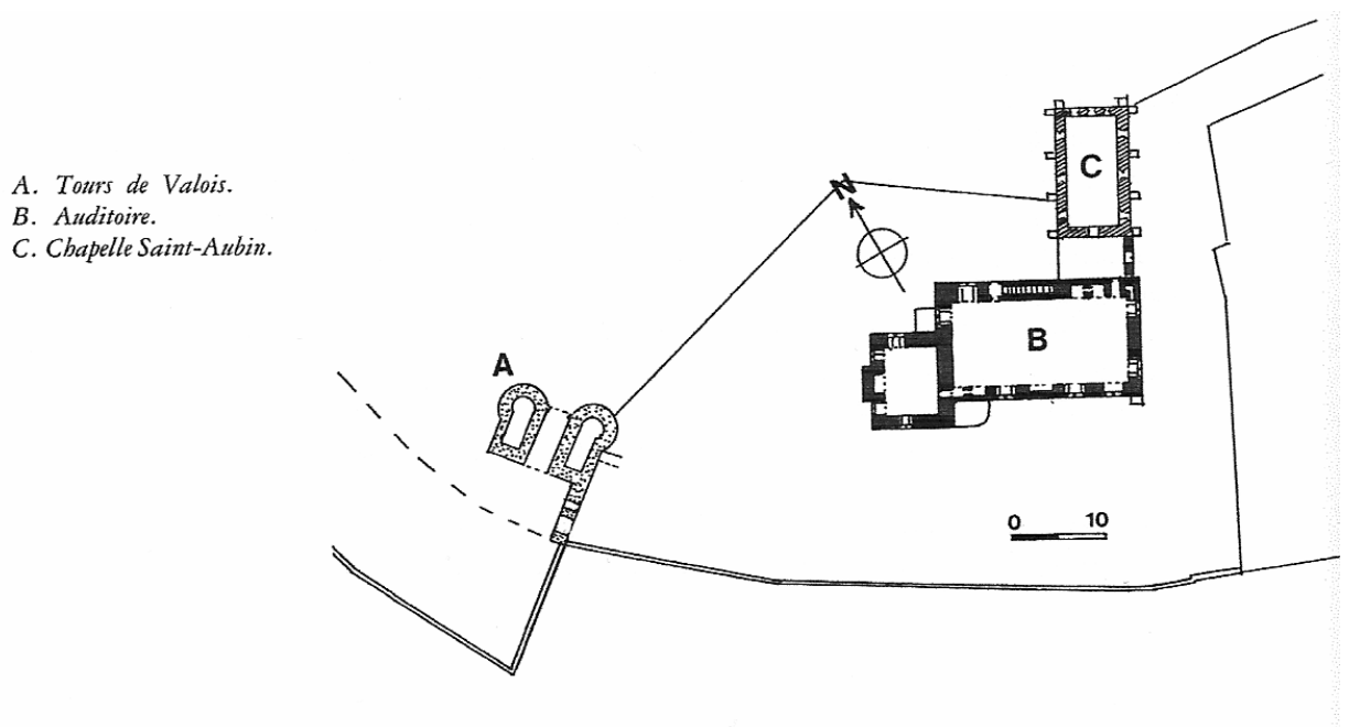
4. Plan général du château de Crépy-en-Valois, illustration tirée de Île-de-France gothique 2, Les demeures seigneuriales par J. Mesqui, Paris, 1988, p. 160
