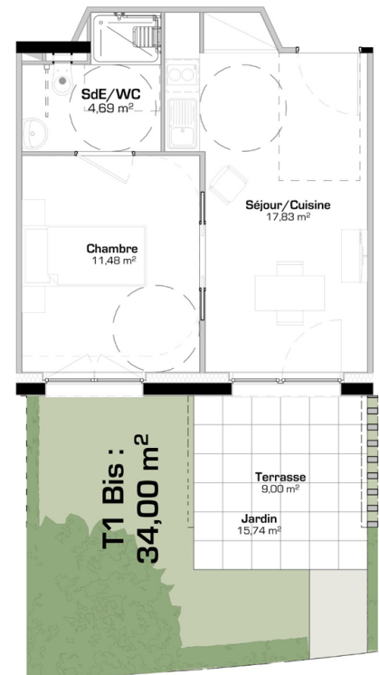
Plan type d'un logement orienté Sud
