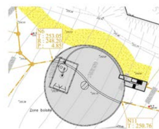
Schéma de principe du futur bassin
