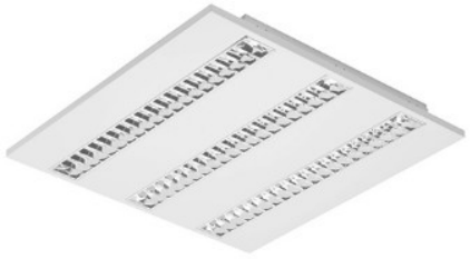
Puissance: 27W 2 circuits d'allumage
