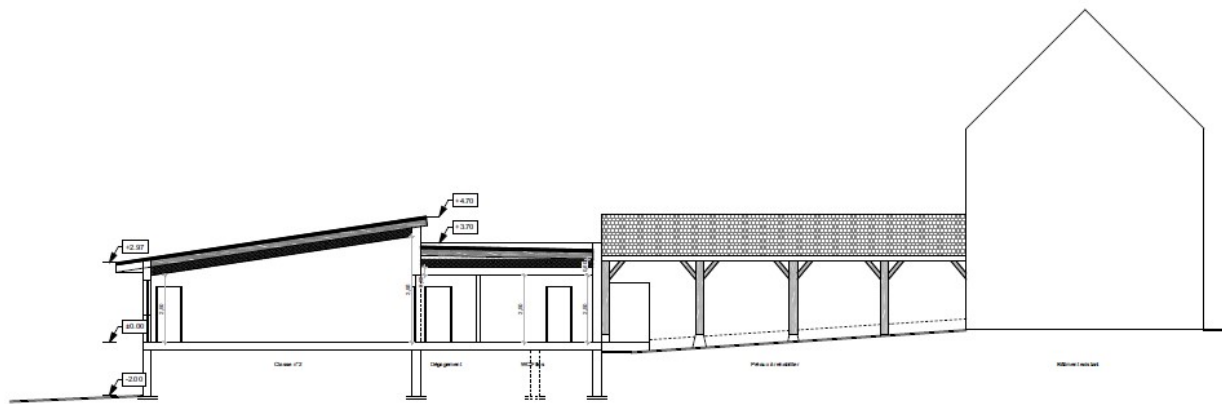
Coupe AA Etat futur
