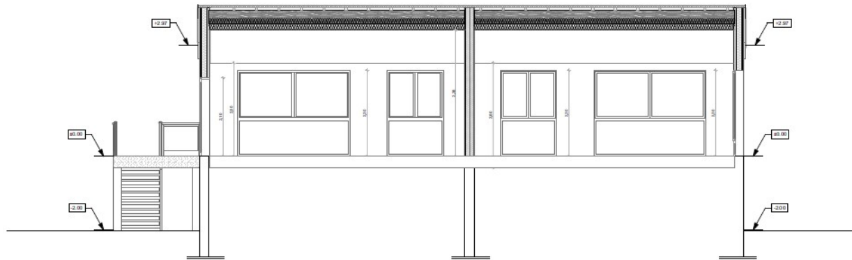
Coupe BB Etat futur
