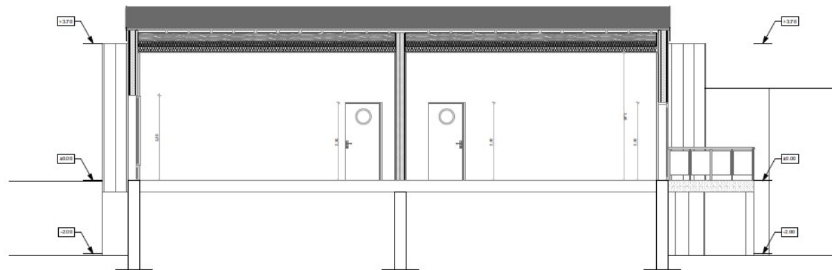
Coupe CC Etat futur
