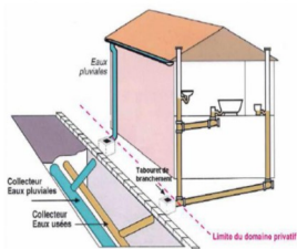
Branchement d'une habitation à un réseau de collecte séparatif
