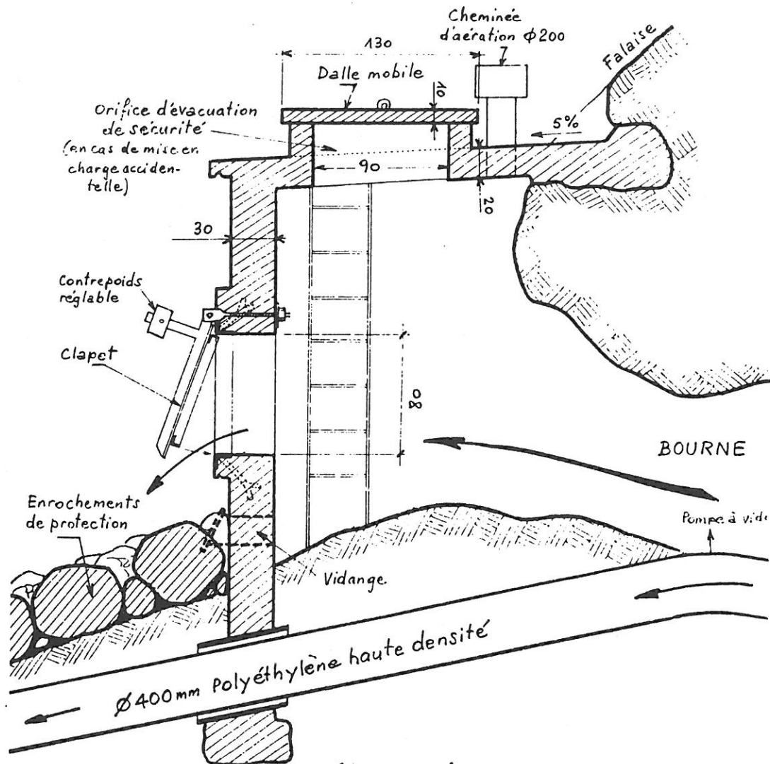
BOURNE - SCHEMA DE L'OUVRAGE DE CAPTAGE
