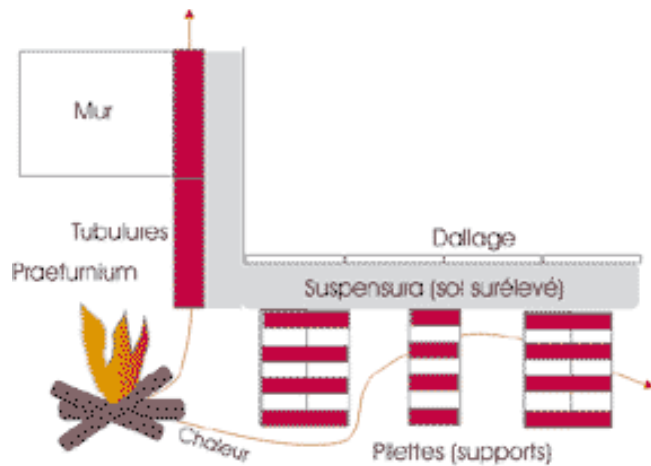
Coupe d'un hypocauste. Dessin d'après JP Adam 1994
