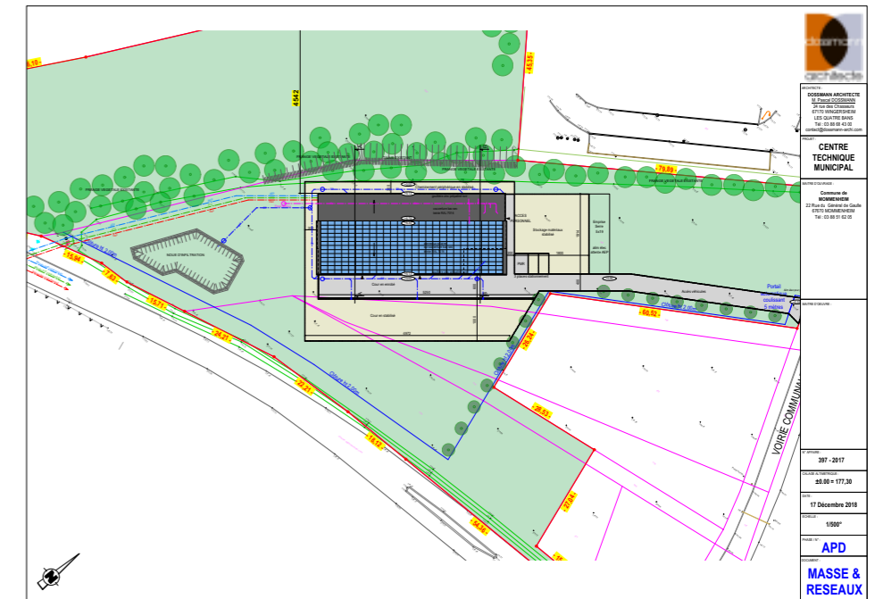
Centre Technique Municipal - Plan de masse provisoire
