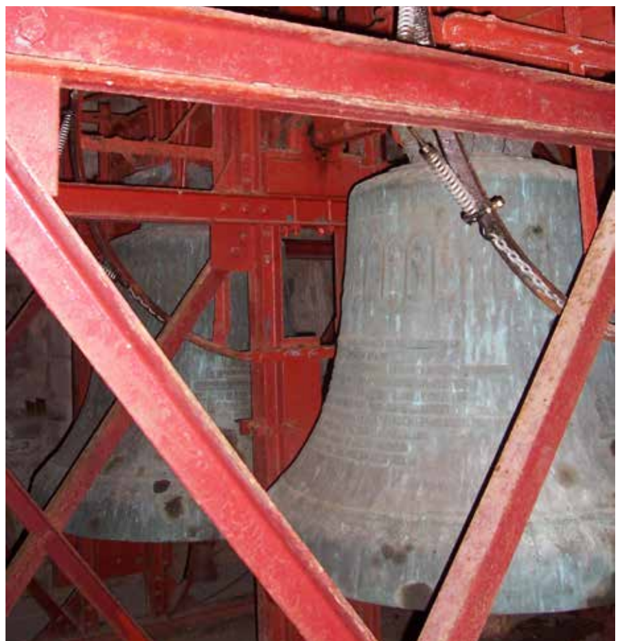
Le beffroi métallique de 1932
